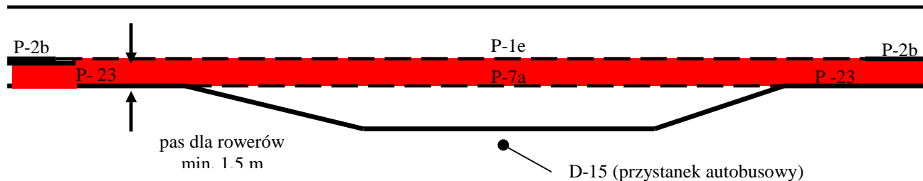
Rys. 31 Zalecane prowadzenie pasa dla rowerów na jezdni z zatoką przystankową.
