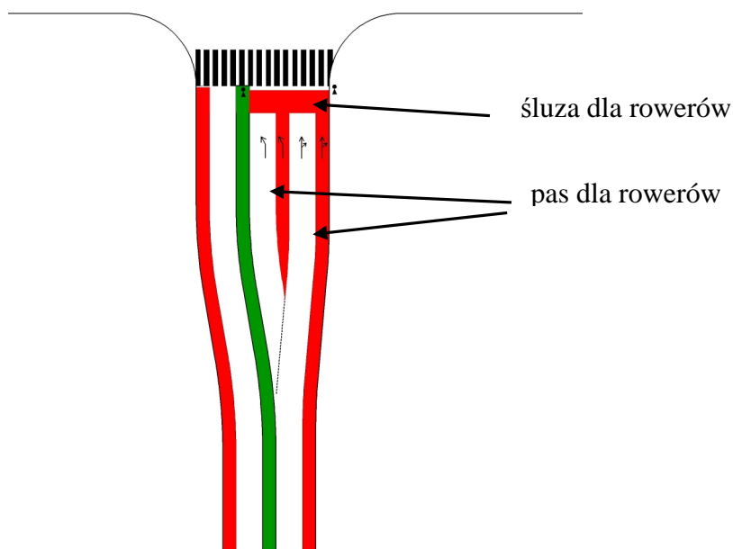
Rys. 21 Przykład rozwiązania wlotu na skrzyżowanie z ruchem rowerowym prowadzonym w jezdni, z zastosowaniem służy dla ruchu rowerowego i wydzielonych pasów do skrętu w lewo.
